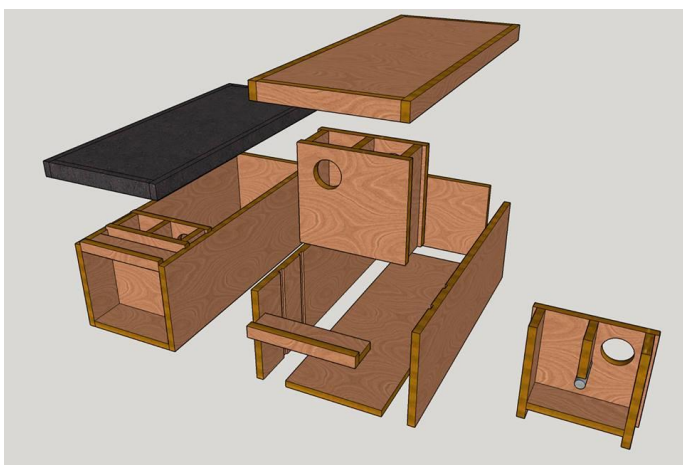
21: Opbouw nestkast
