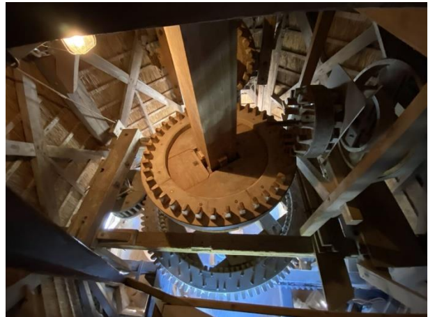
9: Binnenwerk molen Diever
